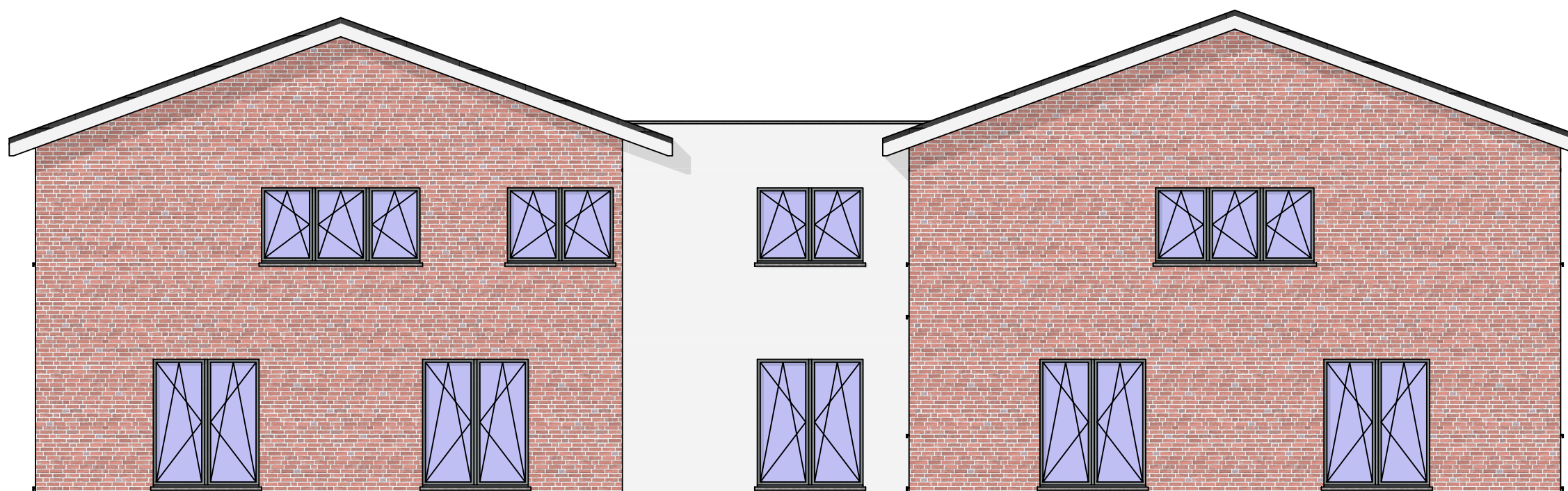
Westansicht
